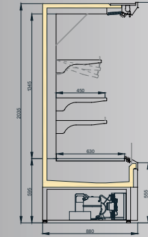
LISTER MT/F&V 900/H2050
