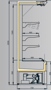
LISTER MT/F&V 750/H2050
