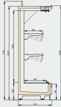
VINSON MT/F&V 750/H2050
