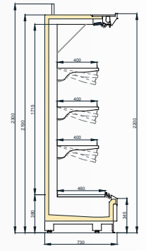
VINSON MT/F&V 750/H2200
