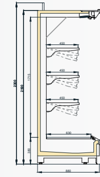
VINSON MT/F&V 900/H2200
