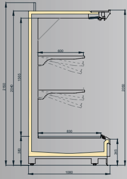
VINSON MT/F&V 1100/H2050
