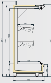
VINSON MT/F&V 900/H2050
