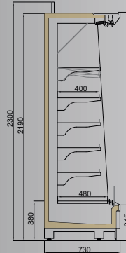
VINSON MT/FV 750/H2200
