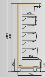
VINSON DP 750/H2050
