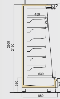
VINSON DP 900/H2200
