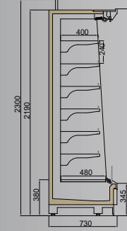
VINSON DP 750/H2200
