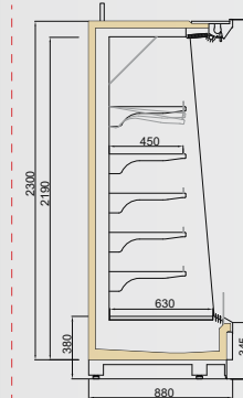
VINSON MT/FV 900/H2200
