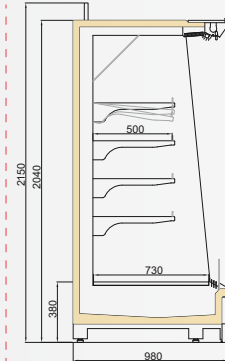
VINSON MT/FV 1000/H2050
