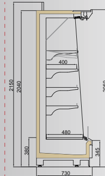
VINSON MT/FV 750/H2050
