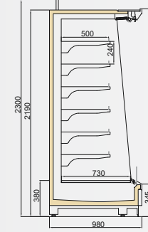
VINSON DP 1000/H2200
