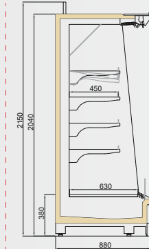
VINSON MT/FV 900/H2050
