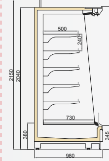
VINSON DP 1000/H2050
