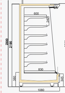
VINSON DP 1100/H2200
