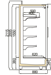
VINSON SLD V1 900/H2050
