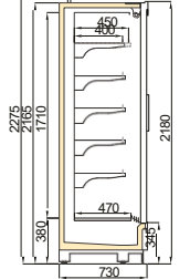
VINSON SLD V1 750/H2200
