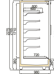
VINSON SLD V1 1000/H2200
