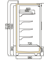
VINSON SLD V1 1000/H2050
