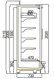
VINSON SLD V1 750/H2050
