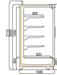
VINSON V1 SLD 1100/H2050
