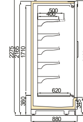
VINSON SLD V1 900/H2200
