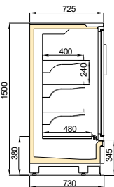
TAKAHE BOX VNZ 750/H1500
