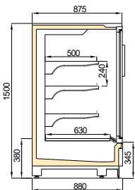
TAKAHE BOX VNZ 900/H1500
