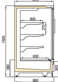
TAKAHE BOX VNZ 900/H1600
