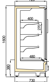
TAKAHE BOX VNZ 750/H1600
