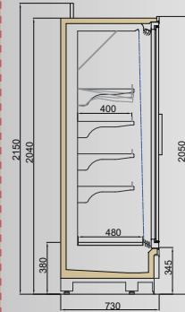
VINSON MT DGD/VNZ 750/H2050
