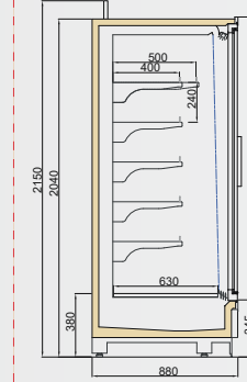
VINSON DGD/VWL 900/H2050
