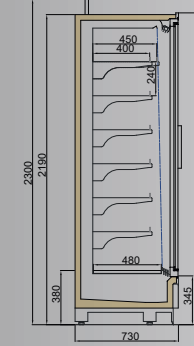
VINSON DGD/VNZ 750/H2200
