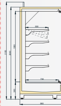
VINSON MT DGD/T55 1000/H2050
