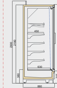
VINSON MT DGD/VNZ 900/H2200
