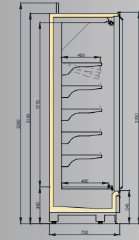
VINSON MT DGD/T55 750/H2200
