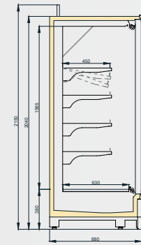
VINSON MT DGD/T55 900/H2050
