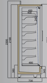
VINSON DGD/TKY 750/H2200
