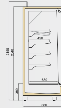
VINSON MT DGD/TKY 900/H2050
