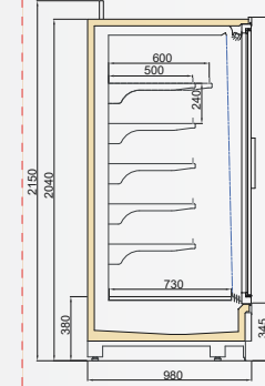
VINSON DGD/VWL 1000/H2050
