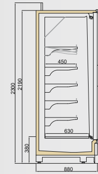
VINSON MT DGD/TKY 900/H2200
