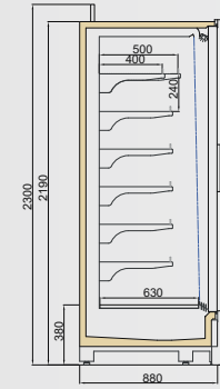
VINSON DGD/TKY 900/H2200
