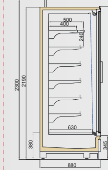
VINSON DGD/VNZ 900/H2200
