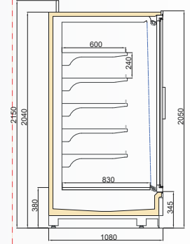
VINSON DGD/VWL 1100/H2050
