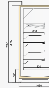
VINSON MT DGD/TKY 1100/H2200
