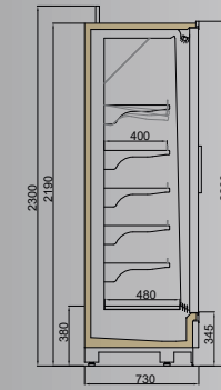
VINSON MT DGD/TKY 750/H2200
