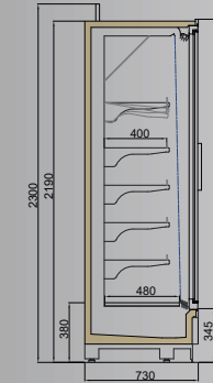
VINSON MT DGD/VNZ 750/H2200
