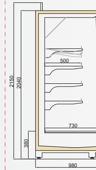
VINSON MT DGD/TKY 1000/H2050
