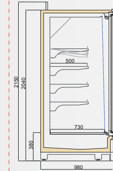
VINSON MT DGD/VWL 1000/H2050
