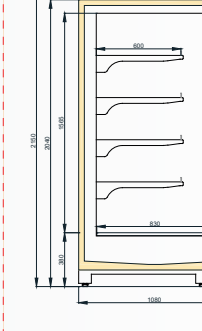
VINSON DGD/T55 1100/H2050
