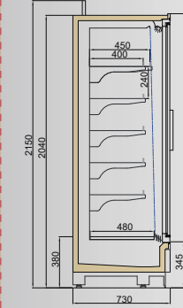
VINSON DGD/VWL 750/H2050
