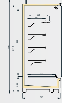
VINSON DGD/T55 900/H2050
