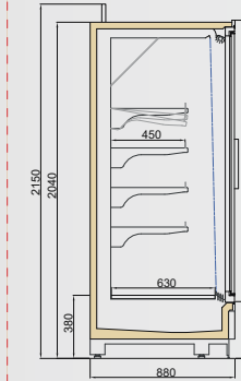
VINSON MT DGD/VWL 900/H2050
