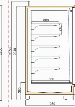
VINSON DGD/TKY 1100/H2050
