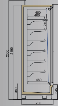
VINSON DGD/VWL 750/H2200
