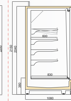
VINSON MT DGD/TKY 1100/H2050
