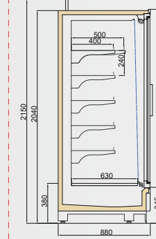
VINSON DGD/VNZ 900/H2050
