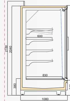
VINSON MT DGD/VNZ 1100/H2050
