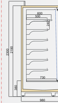
VINSON DGD/TKY 1000/H2200
