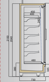
VINSON DGD/VNZ 750/H2050
