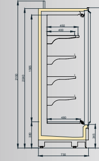
VINSON DGD/T55 750/H2050
