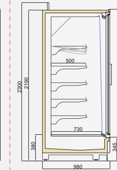
VINSON MT DGD/VNZ 1000/H2200
