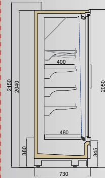
VINSON MT DGD/VWL 750/H2050
