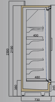
VINSON MT DGD/VWL 750/H2200
