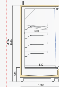
VINSON MT DGD/VWL 1100/H2050
