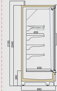
VINSON MT DGD/VNZ 900/H2050
