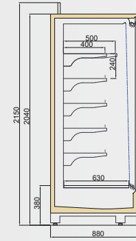
VINSON DGD/TKY 900/H2050
