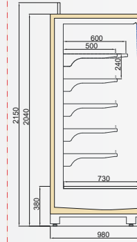
VINSON DGD/TKY 1000/H2050
