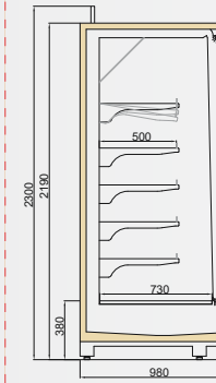
VINSON MT DGD/TKY 1000/H2200
