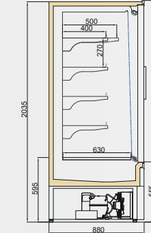
LISTER DGD/TKY 900/H2050
