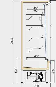
LISTER DGD/TKY 750/H2050
