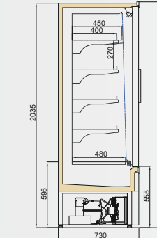
LISTER DGD/TKY 750/H2050
