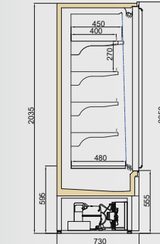
LISTER DGD/T55 750/H2050
