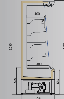
LISTER DP 750/H2050
