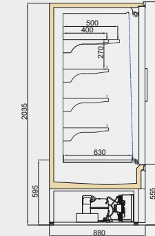
LISTER DGD/TKY 900/H2050
