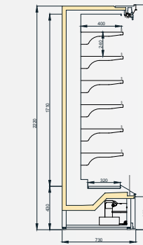
MARAS DP PLUS 750/H2200
