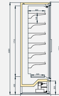
MARAS VWL 750/H2200
