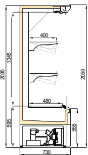
LISTER MT/F&V 750/H2050
