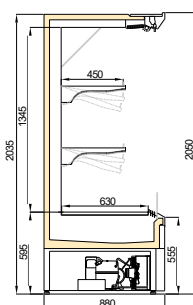
LISTER MT/F&V 900/H2050
