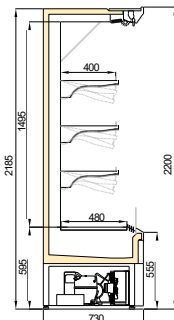
LISTER MT/F&V 750/H2200
