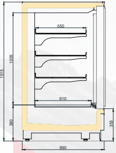
EREBUS BOX T80 900/H1500
