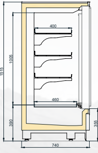
EREBUS BOX T80 750/H1500
