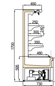
VERNE DP 750/H1700
