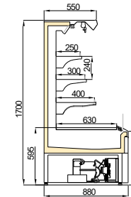
VERNE DP 900/H1700
