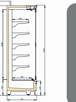
VINSON SGD 750/H2200
