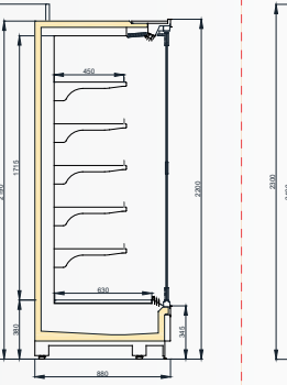
VINSON SGD 900/H2200
