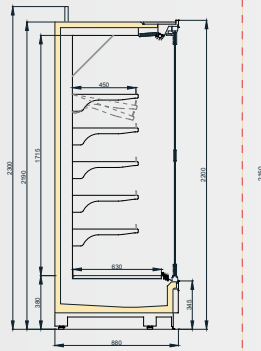
VINSON MT DGD/SGD 900/H2200
