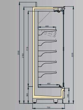
VINSON MT DGD/SGD 750/H2200
