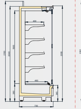
VINSON SGD 750/H2050
