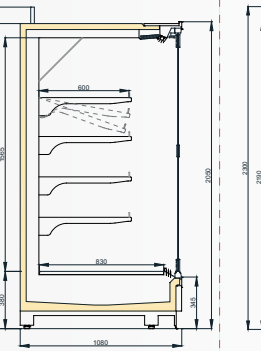
VINSON MT DGD/SGD 1100/H2050
