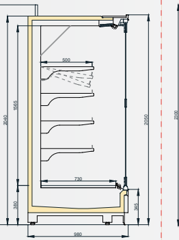
VINSON MT DGD/SGD 1000/H2050
