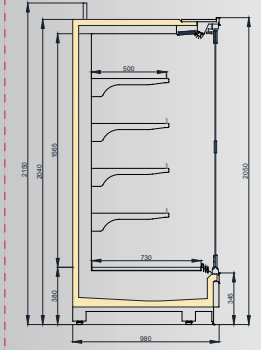
VINSON SGD 1000/H2050
