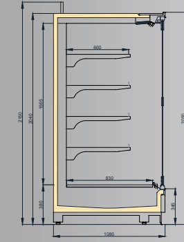
VINSON SGD 1100/H2050
