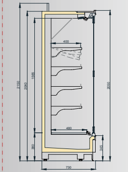
VINSON MT DGD/SGD 750/H2050
