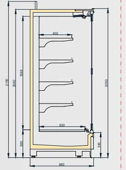
VINSON SGD 900/H2050
