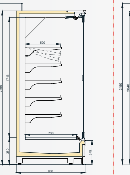
VINSON MT DGD/SGD 1000/H2200
