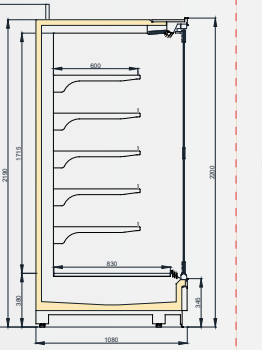
VINSON SGD 1100/H2200
