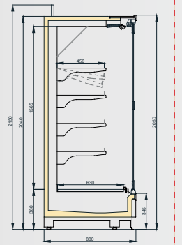
VINSON MT DGD/SGD 900/H2050
