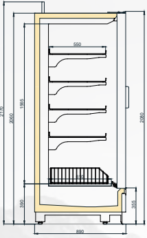
FOSTER SKY 900/H2050
