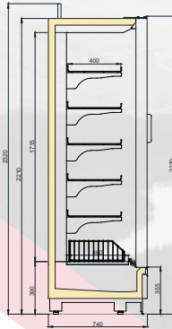
FOSTER SKY 750/H2200
