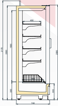
FOSTER SKY 750/H2050
