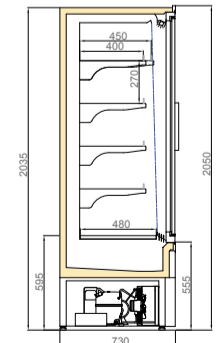
LISTER DGD/VWL 750/H2050
