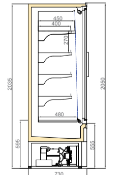
LISTER DGD/VNZ 750/H2050
