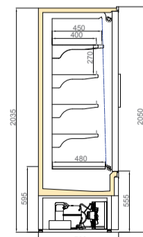
LISTER DGD/TKY 750/H2050
