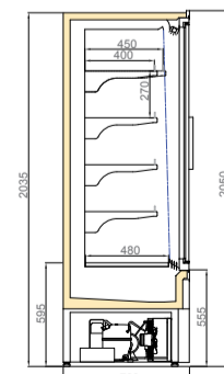
LISTER DGD/VWL 750/H2050
