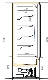
LISTER DGD/T55 750/H2050
