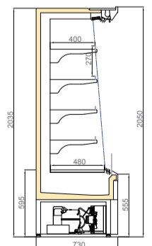
LISTER DP 750/H2050
