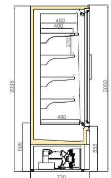
LISTER DGD/VNZ 750/H2050
