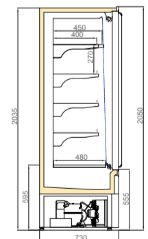
LISTER DGD/T55 750/H2050
