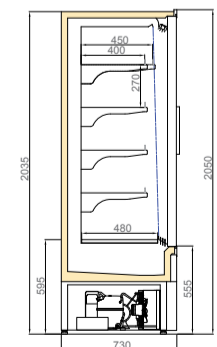
LISTER DGD/TKY 750/H2050
