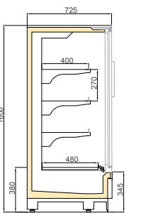
TAKAHE DGD/SKY 750/H1600
