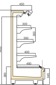
TAKAHE DP 750/H1600
