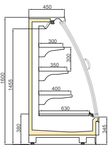
TAKAHE TLD 900/H1600
