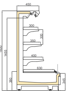
TAKAHE DP 900/H1600
