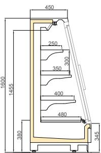
TAKAHE DGD/VNZ 750/H1600
