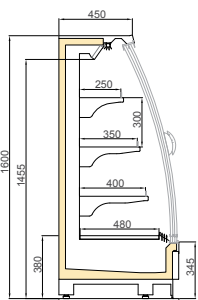
TAKAHE TLD 750/H1600
