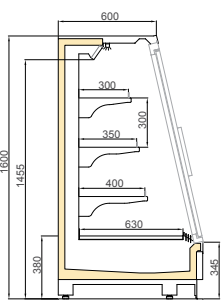
TAKAHE DGD/VNZ 900/H1600
