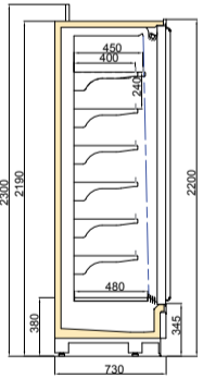
VINSON DGD/T55 750/H2200
