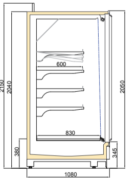
VINSON MT DGD/T55 1100/H2050
