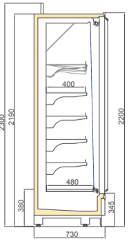
VINSON MT DGD/T55 750/H2200
