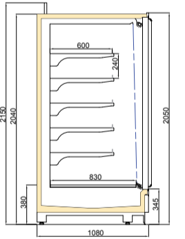
VINSON DGD/T55 1100/H2050
